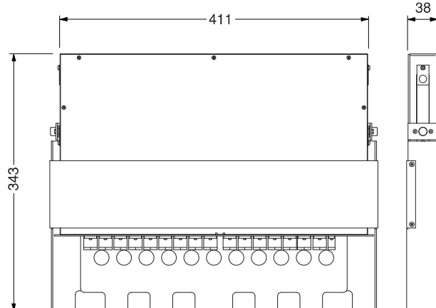
HCOPA32DU2 (スライド構造)
