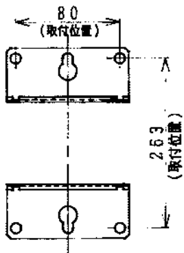
取付寸法
