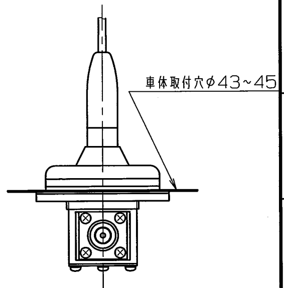
付属品詳細 (1: 3)
