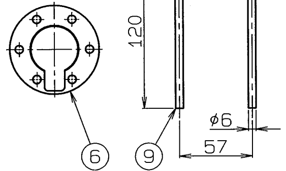
付属品詳細 (1: 3)
