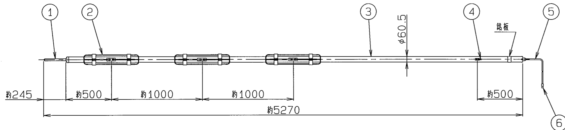
アンテナ外観
