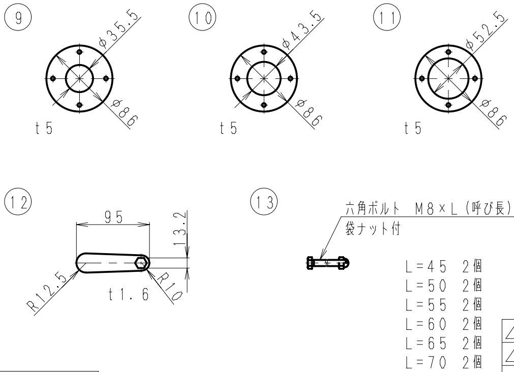
付属品 詳細図 (SCALE 1:5)
