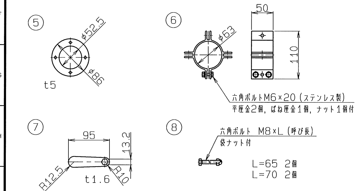
付属品 詳細図 (SCALE 1: 5)
