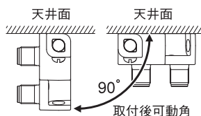
〔天面取付の場合〕
