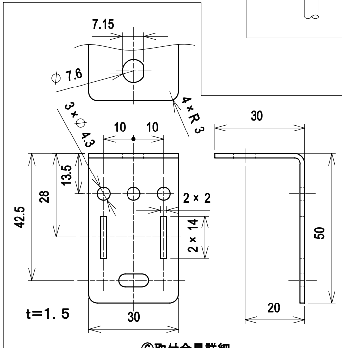
⑥取付金具詳細
