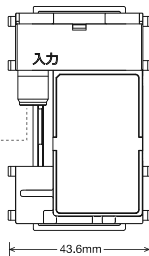
【背面】
