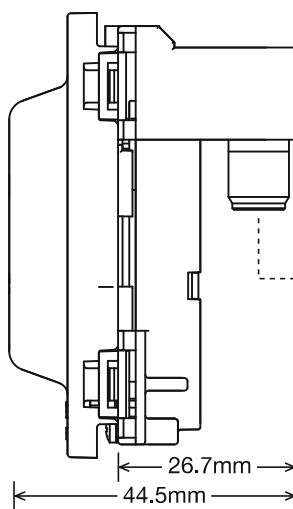
【側面】
