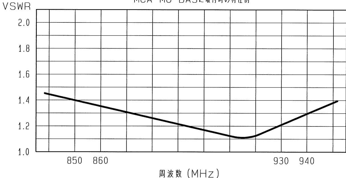
MCA-MG-BA3に取付時の特性例
