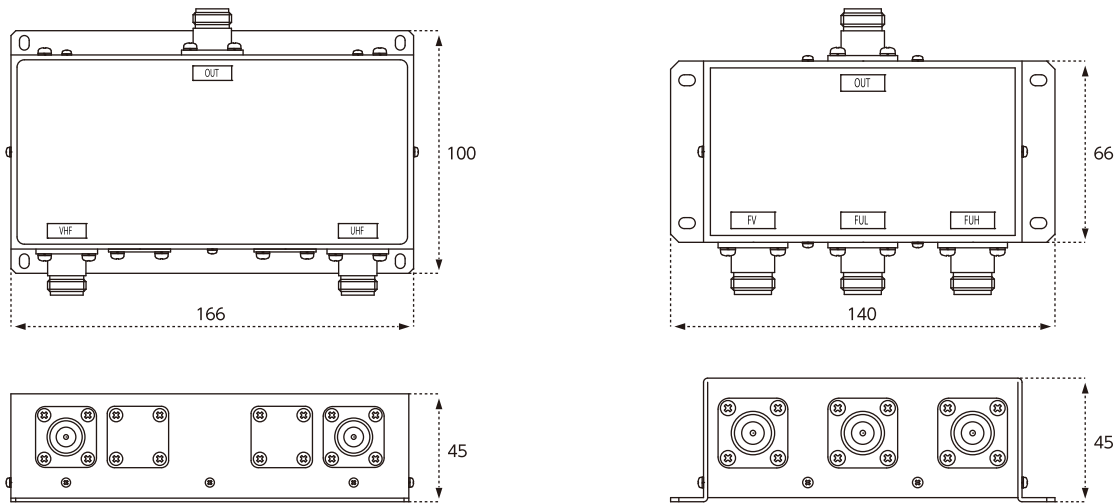
■外觀図
